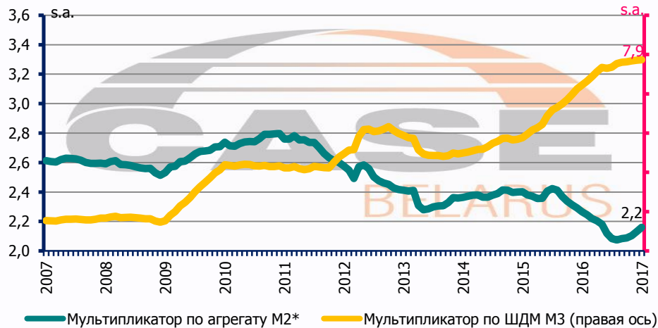
Рис. 3.7 – Денежный мультипликатор
