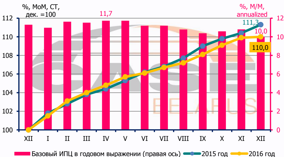
Рис. 1.23 - Базовый ИПЦ
