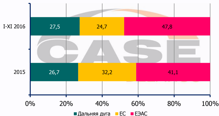
Рис. 5.20 – Диверсификация экспорта
