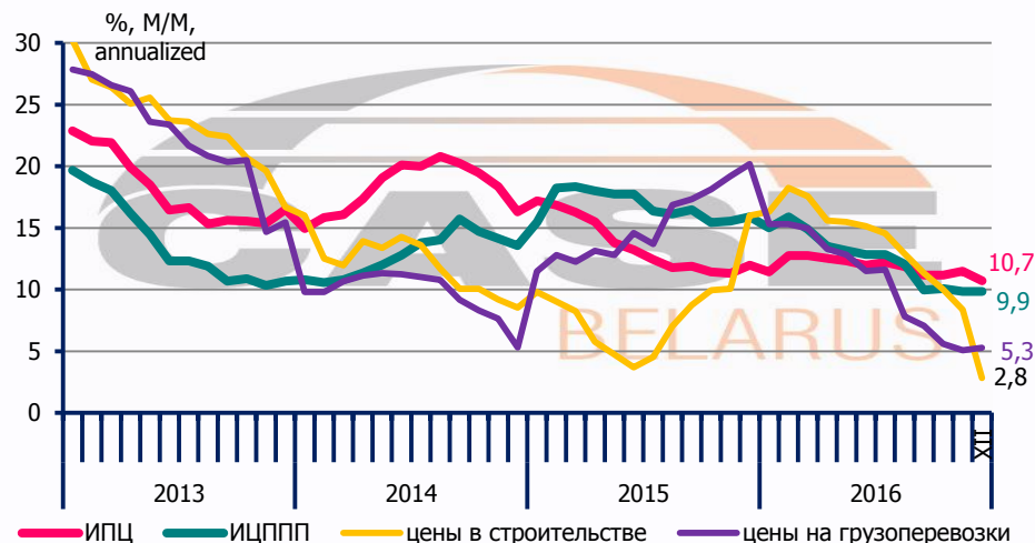
Рис. 1.22 – Индексы цен
