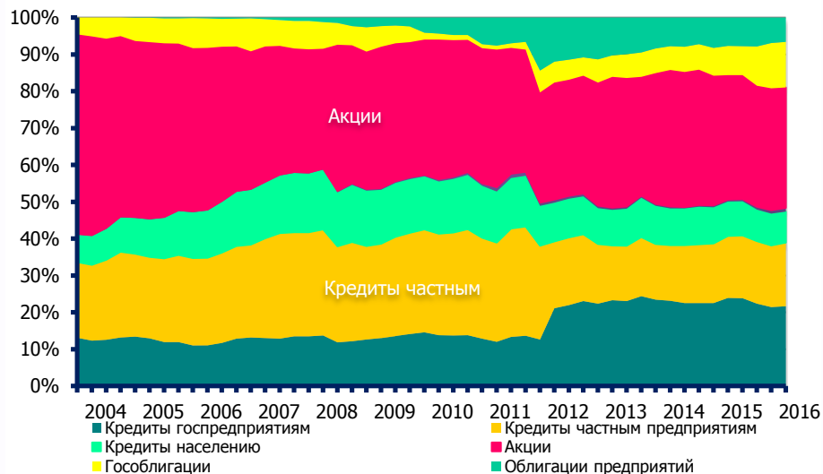
Рис. 3.18 – Структура SDEO
