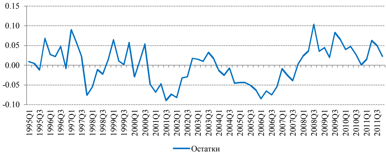
Рис. 2.1. Остатки модели (2.1)
